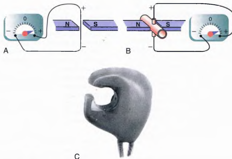
Figura 14-4 Flujómetro de tipo electromagnético en el que se muestra la generación de un voltaje eléctrico en un cable a medida que atraviesa un campo electromagnético (A); generación de un voltaje eléctrico en los electrodos de un vaso sanguíneo cuando el vaso se sitúa en un campo magnético potente y la sangre fluye a través del vaso (B); y una sonda moderna de un flujómetro electromagnético para la implantación crónica alrededor de los vasos sanguíneos (C).
