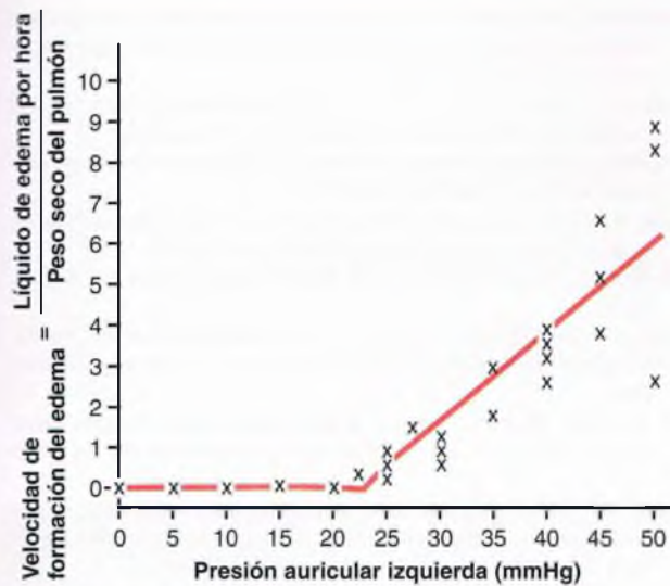
Figura 38-7 Velocidad de pérdida de líquido hacia los tejidos pulmonares cuando aumenta la presión arterial auricular (y la presión capilar pulmonar). (Tomado de Guyton AC, Lindsey AW: Effect of elevated left atrial pressure and decreased plasma protein concentration on the development of pulmonary edema. Circ Res 7:649, 1959.)
