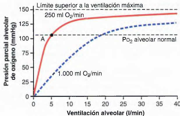
Figura 39-4 Efecto de la ventilación alveolar sobre la P_{O_2} alveolar a dos velocidades de absorción de oxígeno desde los alvéolos: 250 ml/min y 1.000 ml/min. El punto A es el punto operativo normal.
