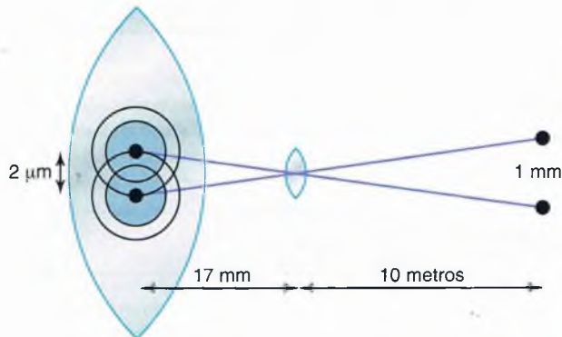
Figura 49-16 Agudeza visual máxima para dos fuentes puntuales de luz.
