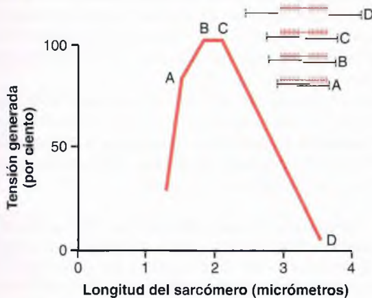
Figura 6-9 Diagrama longitud-tensión de un sarcómero único contraído totalmente, que muestra la máxima fuerza de contracción cuando el sarcómero mide de 2 a 2,2\mu\text{m} de longitud. En la parte superior derecha están las posiciones relativas de los filamentos de actina y miosina a diferentes longitudes del sarcómero desde el punto A al punto D. (Modificado de Gordon AM, Huxley AF, Julian FJ: The length-tension diagram of single vertebrate striated muscle fibers. J Physiol 171:28P, 1964.)
