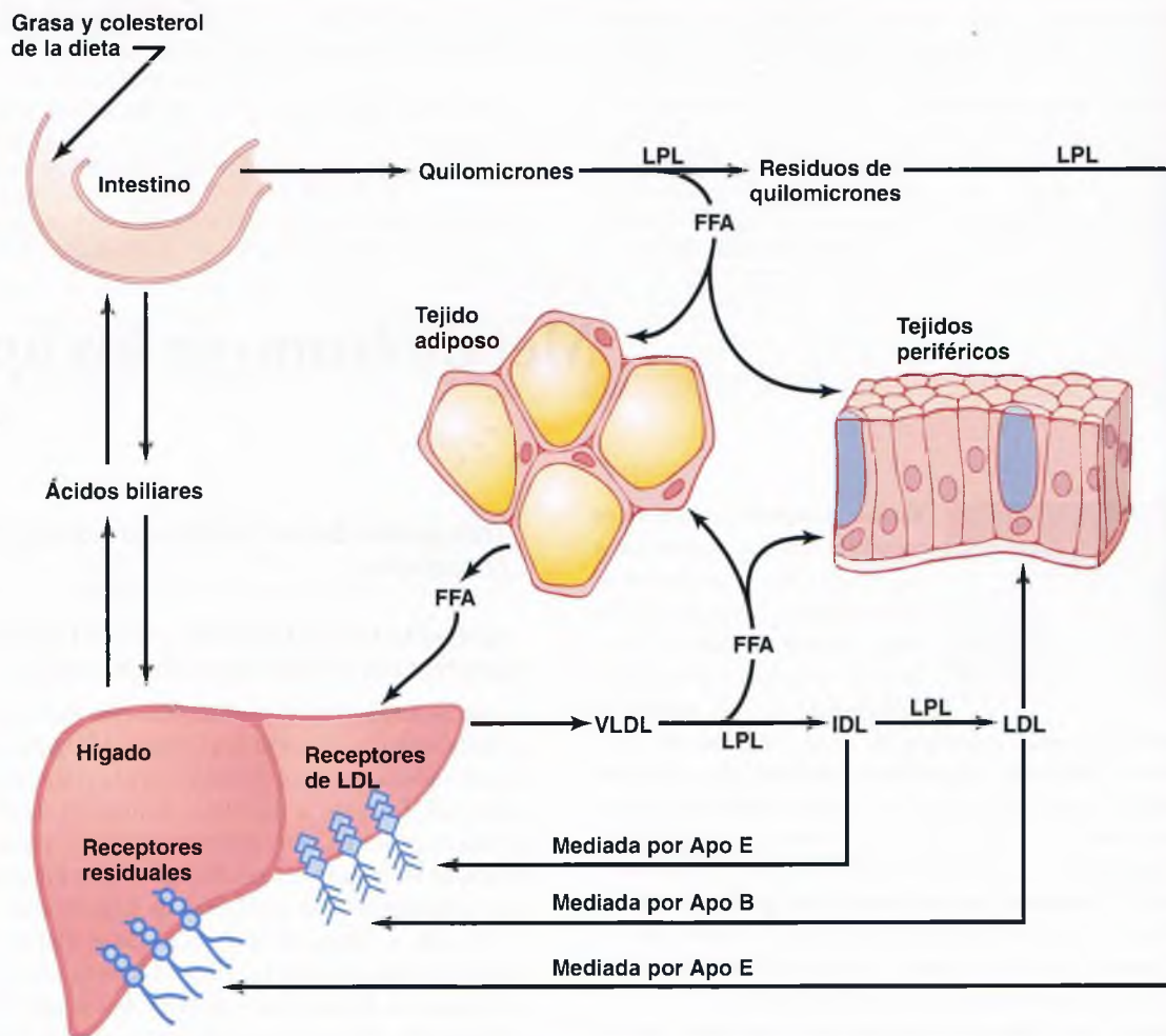
Figura 68-1 Resumen de las rutas principales para el metabolismo de quilomicrones sintetizados en el intestino y de lipoproteínas de muy baja densidad (VLDL) sintetizadas en el hígado. Apo B, apolipoproteína B; Apo E, apolipoproteína E; FFA, ácidos grasos libres; HDL, lipoproteína de alta densidad; IDL, lipoproteína de densidad intermedia; LDL, lipoproteína de baja densidad; LPL; lipoproteína lipasa.
