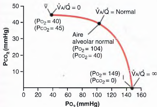
Figura 39-11 Diagrama P_{O_2} - P_{CO_2} , \dot{V}_A/\dot{Q}
